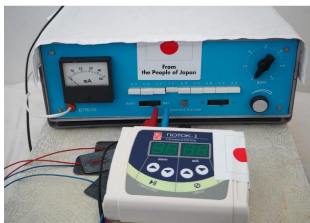
Устройство для диадинамотерапии, предоставленное в рамках проекта. На всех 12 оборудованях есть наклейки, указывающие о поддержке Японии.
